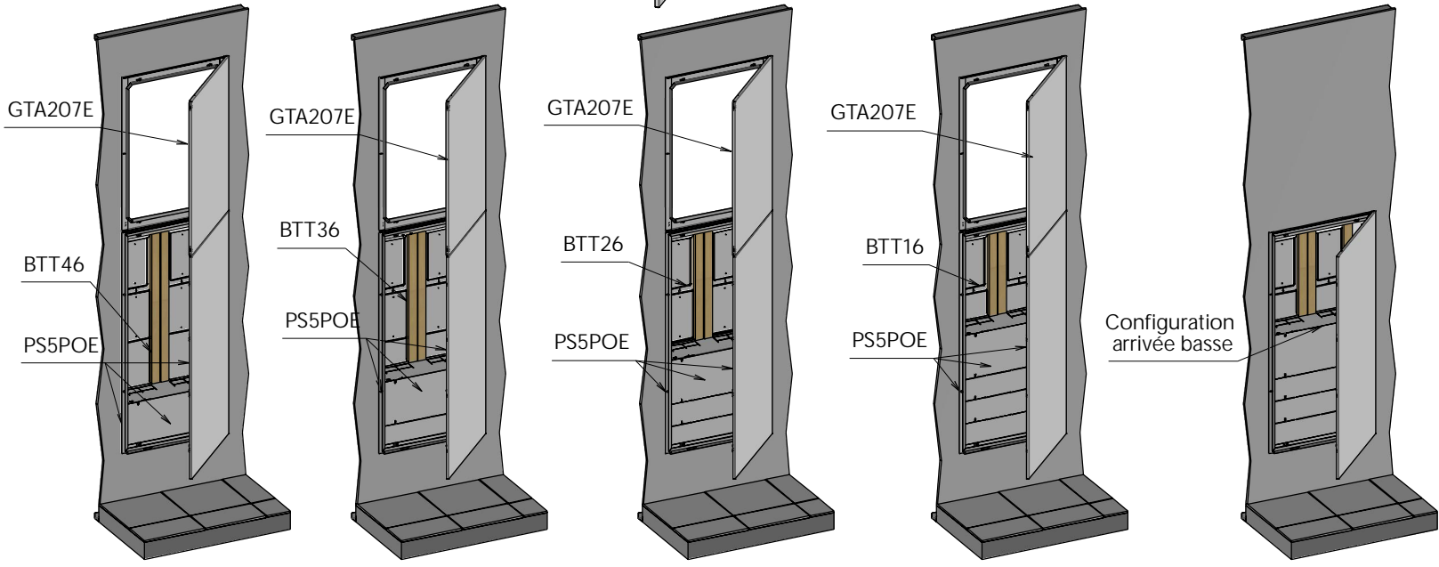
Exemple de mise en oeuvre avec GTA207E
